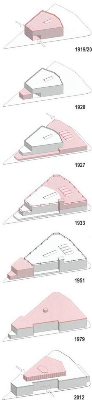
Isometrische Darstellung der Bauphasen. (Zeichnung: raumfindung architekten eth bsa sia, Rapperswil)
